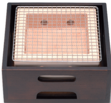
CN-601 火鉢セット(大) 270×270×130 ¥33,000 ●コンロ (CN-601C) 210×210×100 (内160×160×50) ¥15,000 ●木箱 (CN-601F) 内240×240×100 (耐火ボード付) ¥18,000
